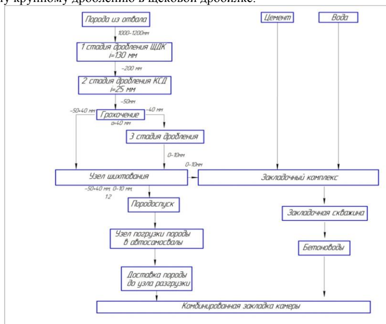
Рис. 2. Технологическая схема подготовки и доставки компонентов комбинированного закладочного массива.
