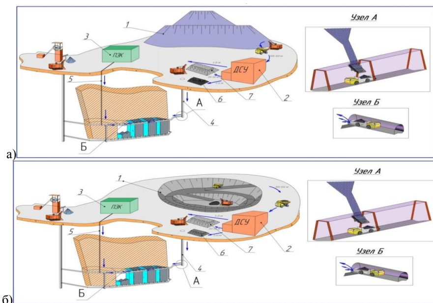
Рис. 1. Принципиальная технологическая схема освоения месторождений: а - доставкой закладочных материалов из отвалов; б - доставкой закладочных материалов из специализированных карьеров. 1 - отвалы пород (а), специализированный карьер по добыче породы (б); 2 - дробильно-сортировочный узел; 3 - поверхностно-закладочный комплекс; 4 - породоспуск; 5 - закладочная скважина; 6 - штабель мелкой фракции; 7 - штабель крупной фракции.
