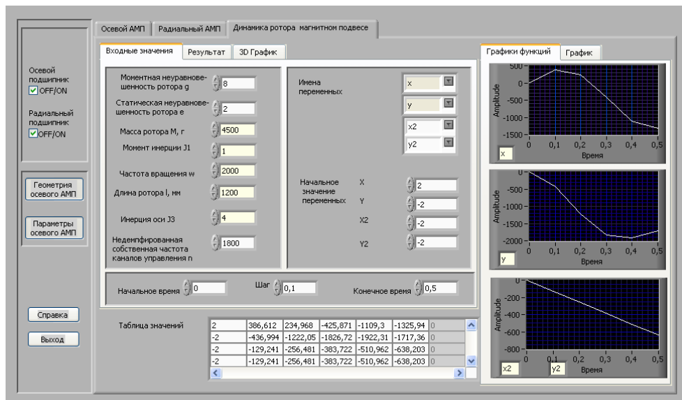
Рисунок 2 - Виртуальный прибор решения дифференциальных уравнений (ввод начальных значений)
