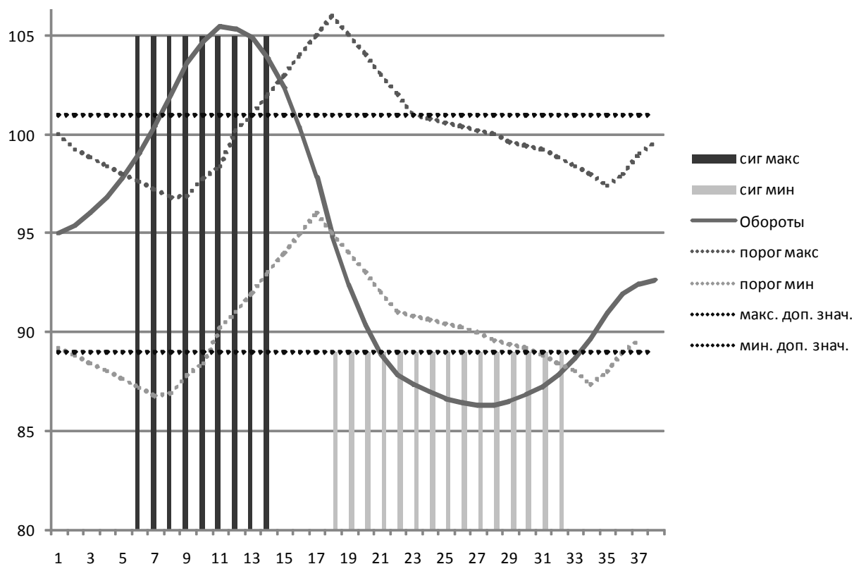
Рисунок 2 - Модель работы сигнализации
