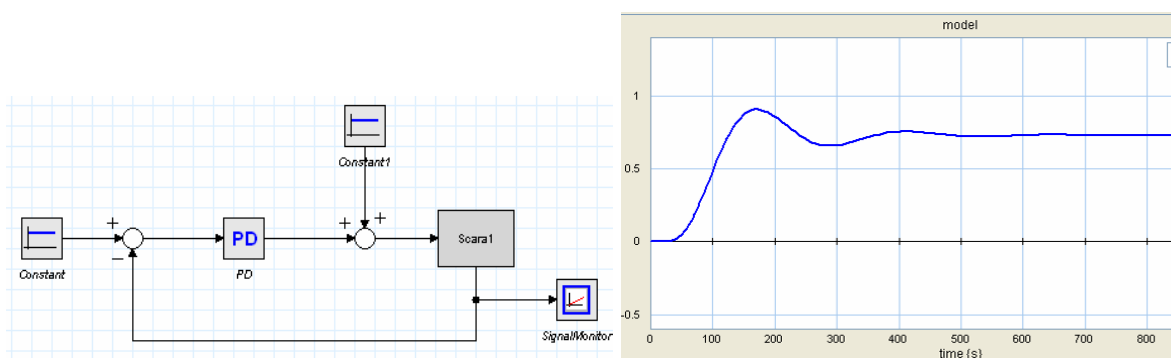
Рисунок 5 - Определение параметров PD-регулятора методом нелинейного программирования
