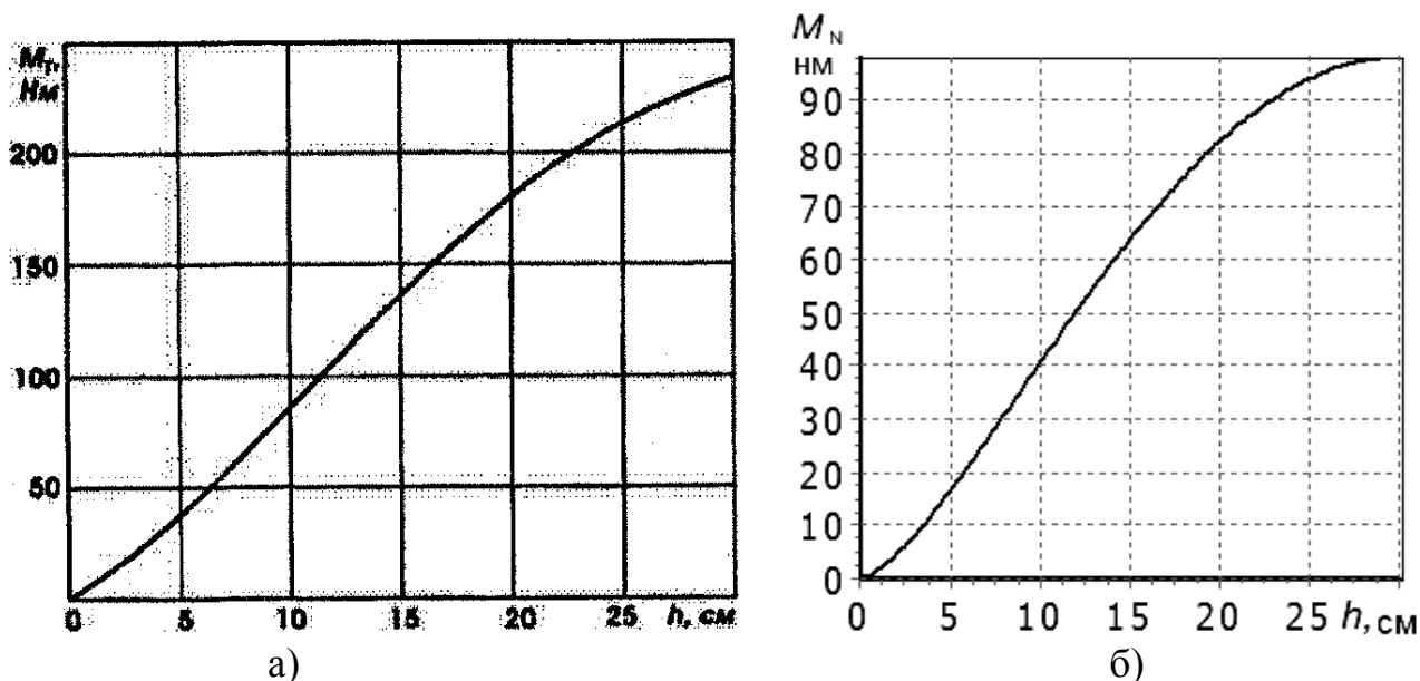
Рисунок 6 – Изменение моментов сопротивления трению от глубины хода рабочего органа-двигателя
