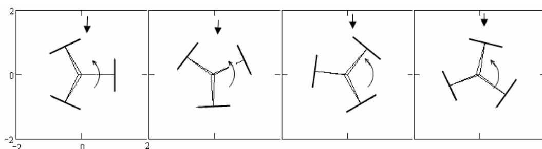
Рисунок 6 - Роторная установка с эксцентриком, который устанавливает необходимый угол атаки крыльев для создания положительного момента
