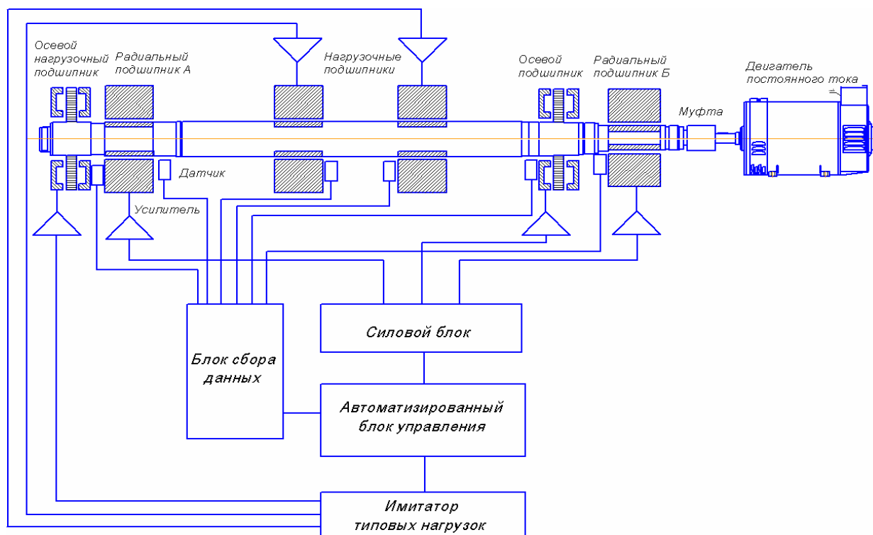
Рисунок 1 - Функциональная схема стенда с возможностью исследовать осевые и радиальные нагрузки
