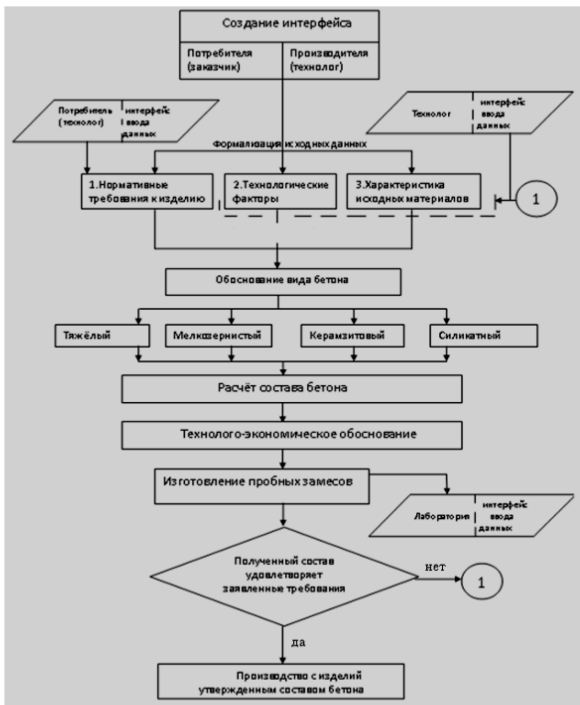
Рисунок 1 - Блок-схема автоматизированной системы по подбору состава бетонных смесей
