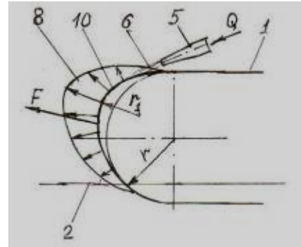
Рисунок 4 - Действие струи на некруглую цилиндрическую поверхность сверху-сзади.
