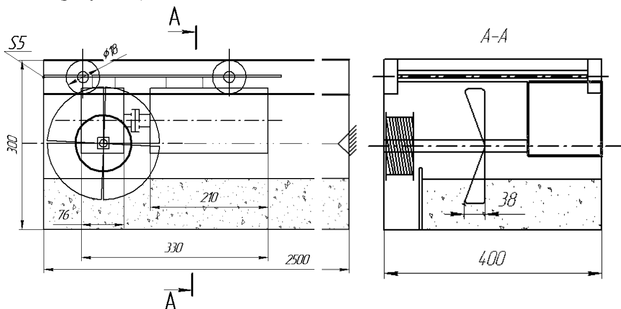
Рисунок 3 – Принципиальная схема почвенного канала
