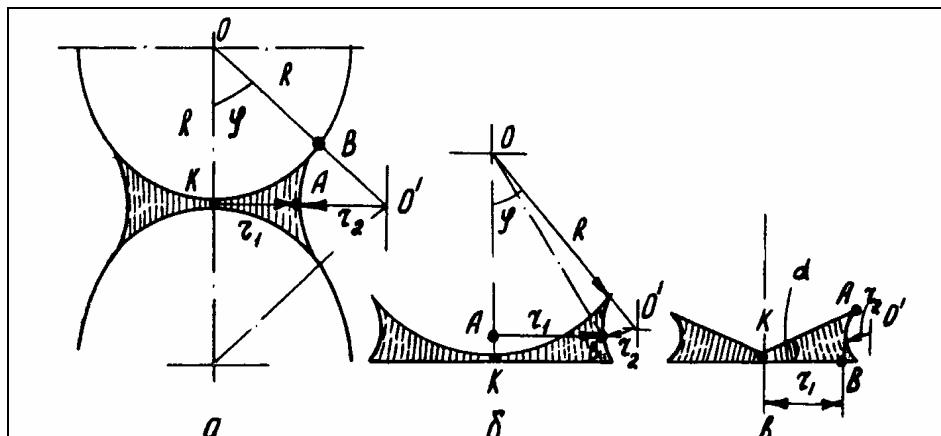
Рисунок 2 - Схема для расчета капиллярного давления и капиллярных сил в зависимости от формы контакта минеральных частиц формовочной смеси:
