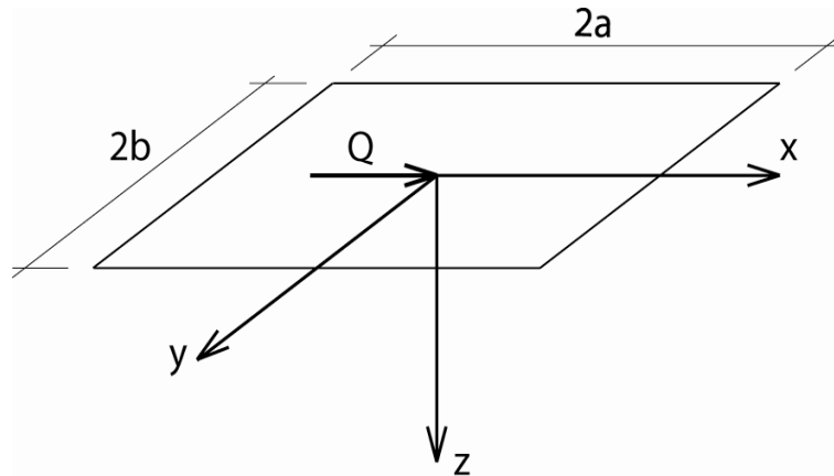
Рисунок 1 - Схема определения вертикальных напряжений от горизонтальной нагрузки
