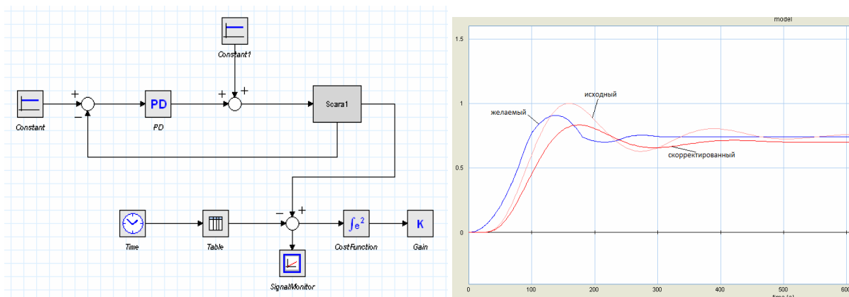
Рисунок 4 - Определение параметров PD-регулятора методом ЗОНИТА
