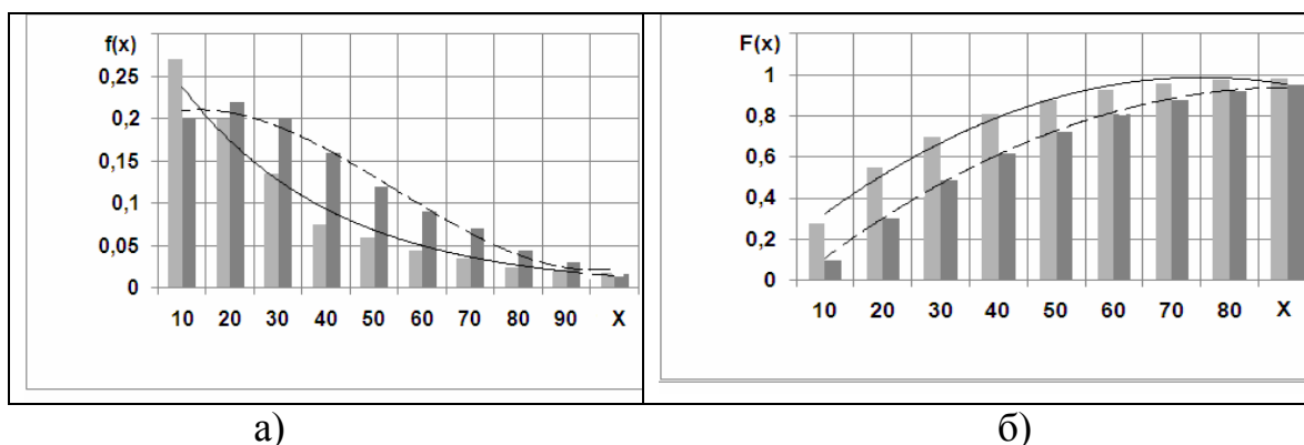
Рисунок 4 - Дифференциальная (а) и интегральная (б) функции распределения следов капель по размерам
