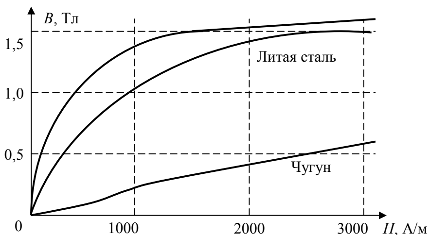
Рисунок 1 - Кривые намагничивания некоторых электротехнических материалов
