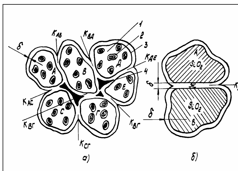
Рисунок 1 - Структура уплотненной фосфатной смеси (а) и схема связи двух кварцевых песчинок (б):
