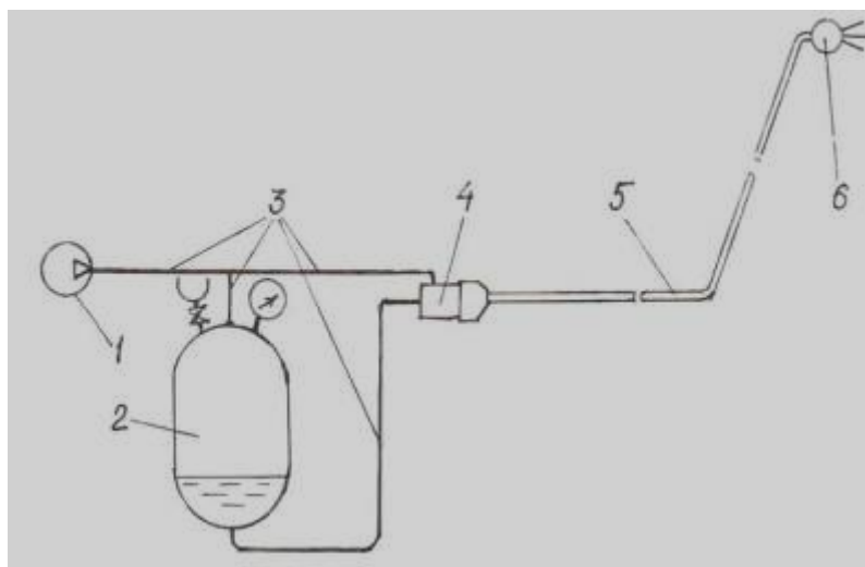
Рисунок 1 - Схема опытной установки
