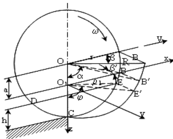
Рисунок 4 – Схема к определению момента сопротивления трения почвы о боковую поверхность эллипсоидной лопасти рабочего органа-двигателя
