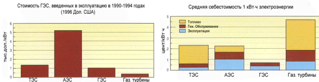
Рисунок 3 - Стоимость ГЭС и средняя себестоимость 1 кВт ч электроэнергии
