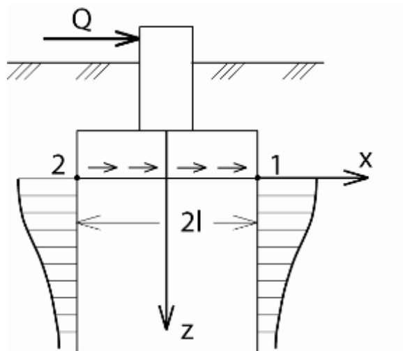
Рисунок 2 - Схема распределения вертикальных напряжений в основании от горизонтальной нагрузки
