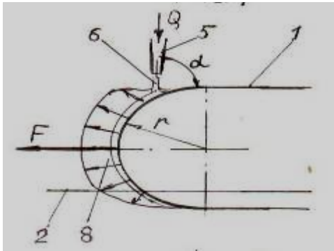
Рисунок 3 - Действие струи на цилиндрическую поверхность сверху-вниз.
