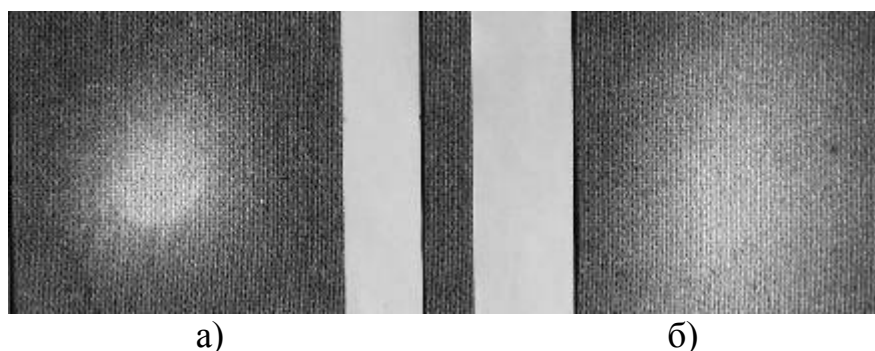
Рисунок 3 – Отпечатки красочного факела при контрольном (а) и опытном (б) вариантах нанесения ЛКМ
