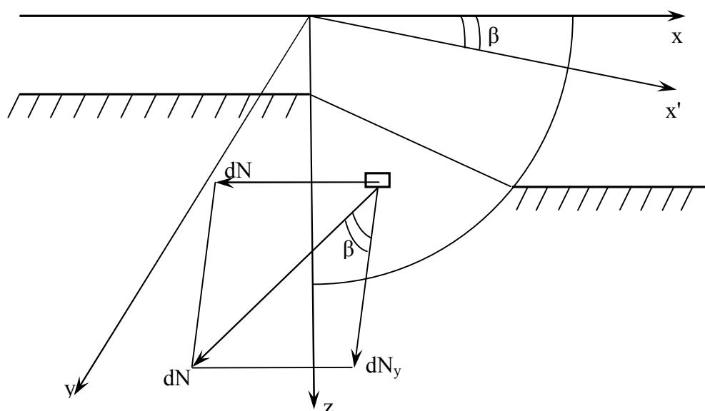
Рисунок 5 – Схема к определению момента сопротивления силы нормальной реакции эллипсовидной лопасти рабочего органа-двигателя
