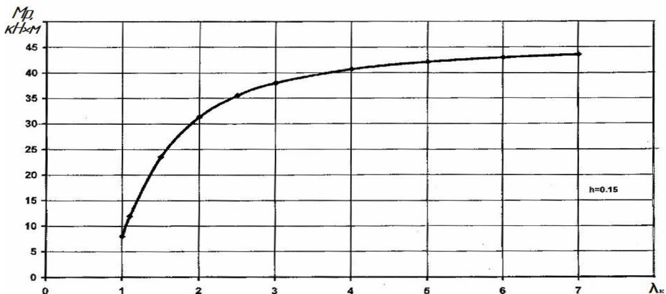
Рисунок 4 - Зависимость момента сопротивления резанию от режима работы рабочего органа-двигателя
