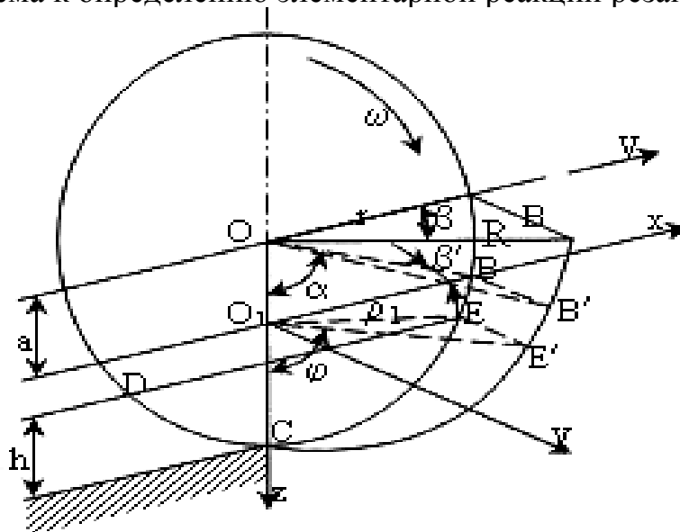
Рисунок 2 – Схема к определению момента сопротивления резанию лезвием эллипсовидной лопасти почвообрабатывающего рабочего органа-двигателя
