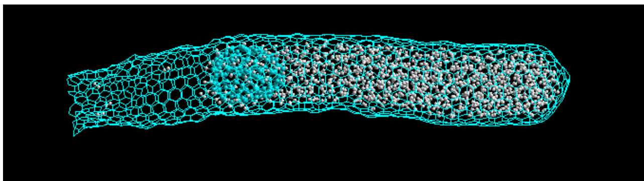
Рисунок 4 - Сжатие молекулярного водорода внутри УНТ фьюззиболлом
