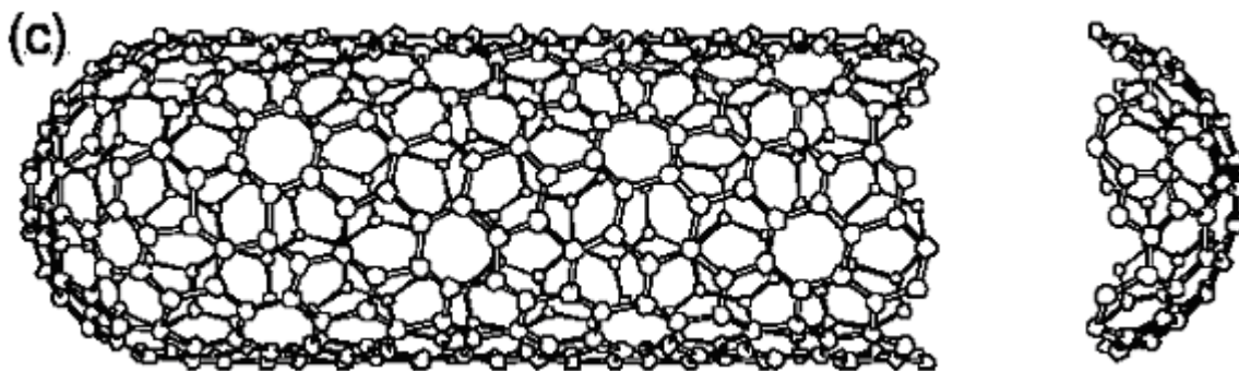
Рисунок 1 - Углеродная нанотрубка и ее «крышка»
