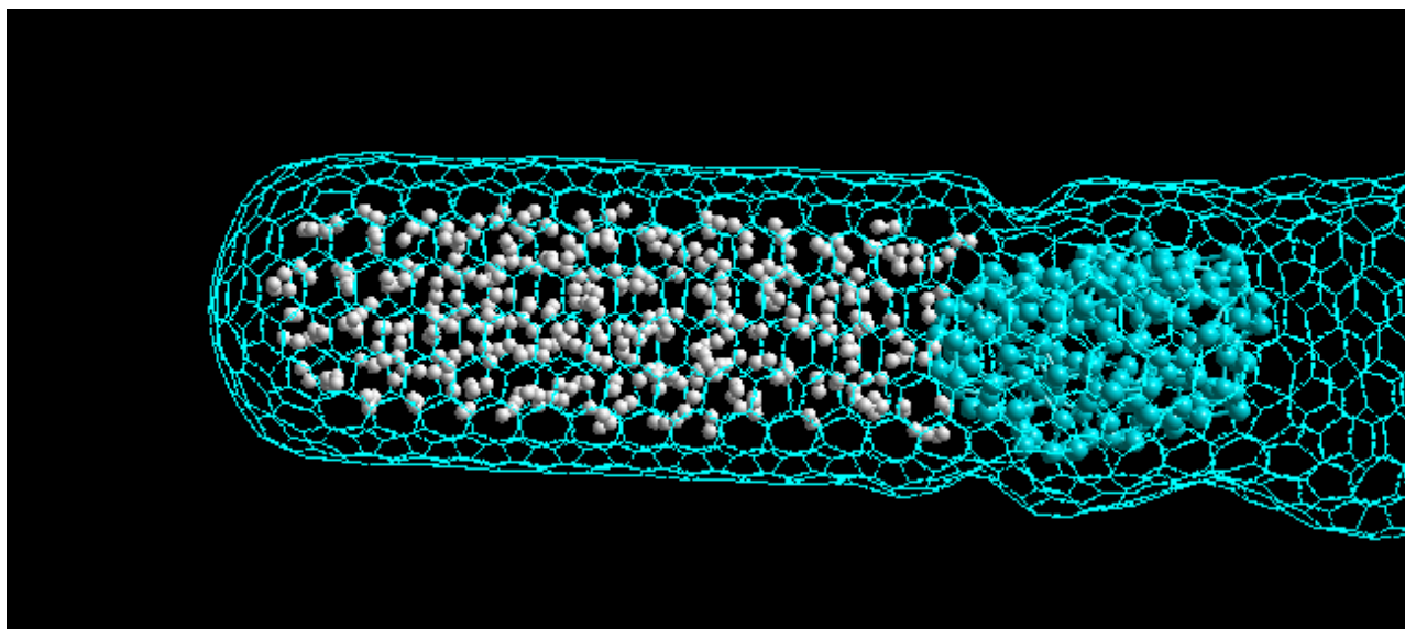
Рисунок 2 - Сжатие водорода фуллереном C_{180} в УНТ (10,10)
