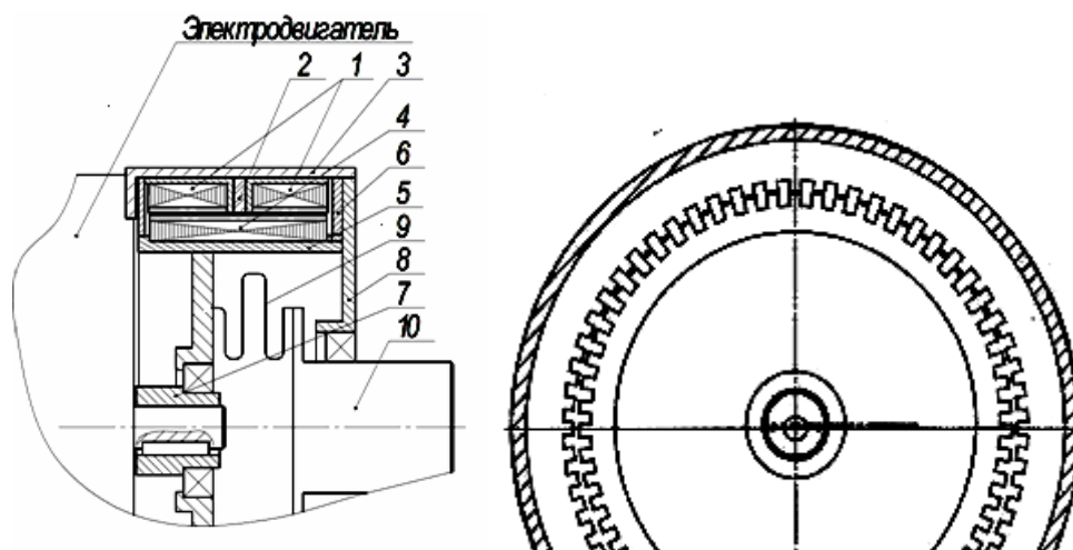
Рисунок 1 - Устройство механической передачи с использованием магнитных сил притяжения
