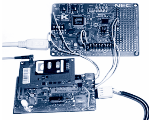
Рисунок 4 - Фотография GSM-модуля подключенного к оценочному комплекту.
