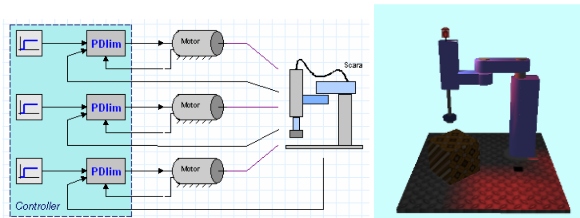
Рисунок 2 -Система позиционирования (программный робот)
