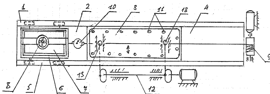
Рисунок 2 - Схема лабораторной установки
