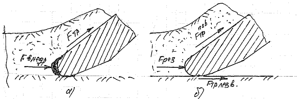
Рисунок 1 - Схемы взаимодействия двухгранного клина с материалом: а – пассивный клин; б – активный клин
