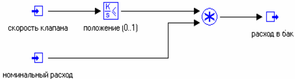
Рисунок 3 - Схема модели клапана
