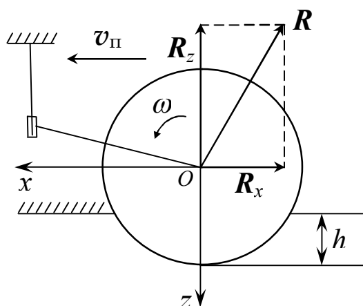
Рисунок 1 - Схема движения диска
