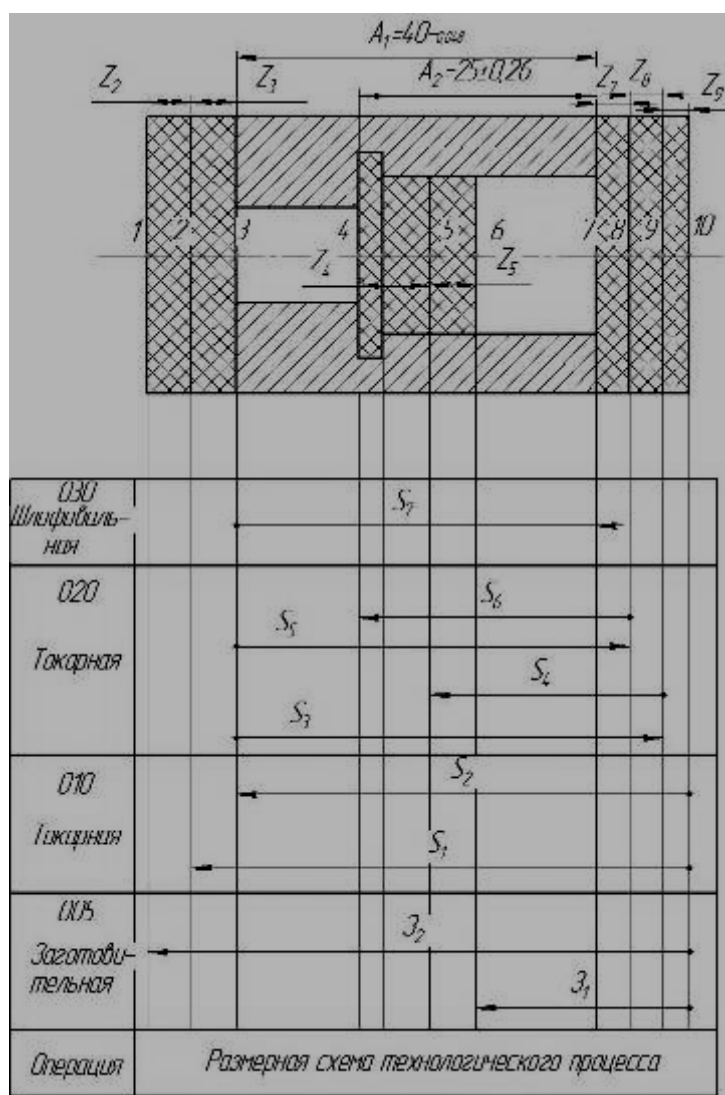
Рисунок 1 - Размерная схема технологического процесса
