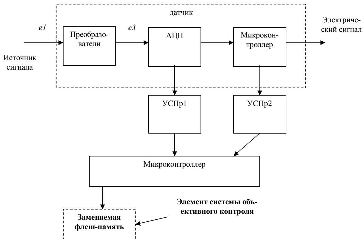
Рисунок 2 - Упрощенная схема интеллектуального датчика
