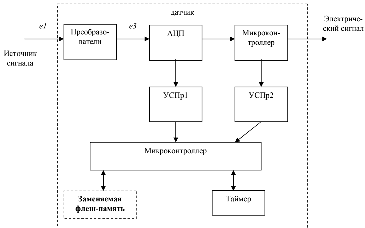
Рисунок 3 - Структурная схема типового интеллектуального датчика
