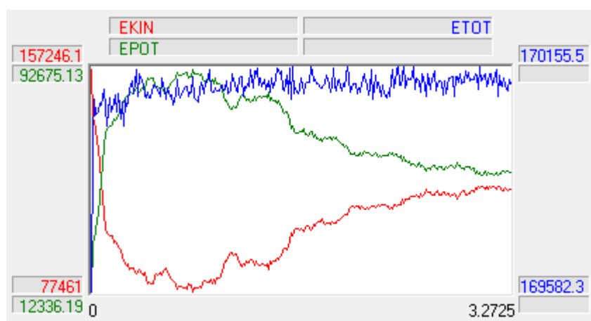
Рисунок 5 - Графики зависимости энергии системы от времени
