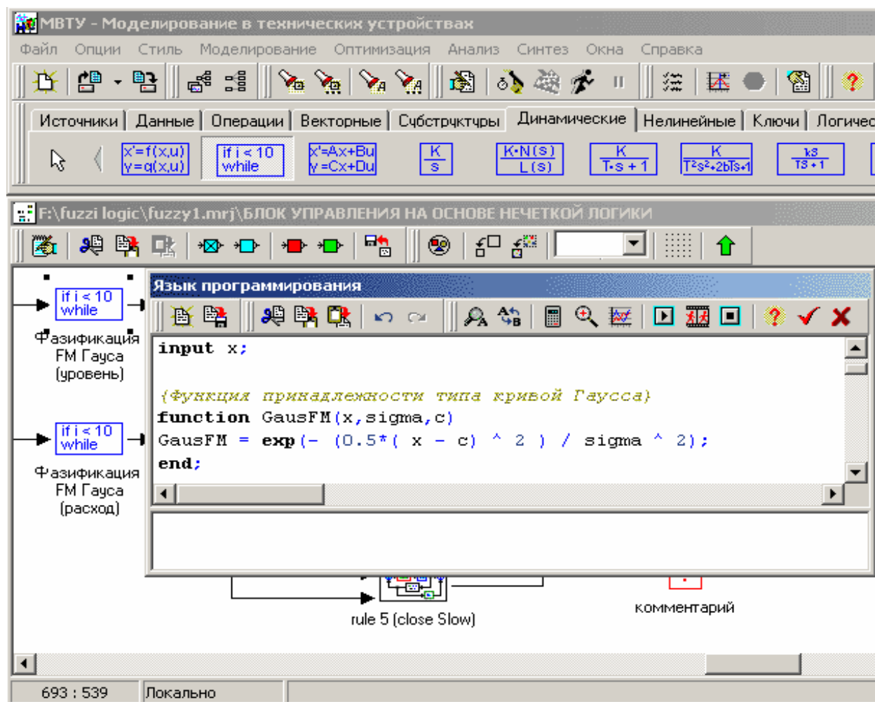
Рисунок 1 - Окно редактора языка программирования
