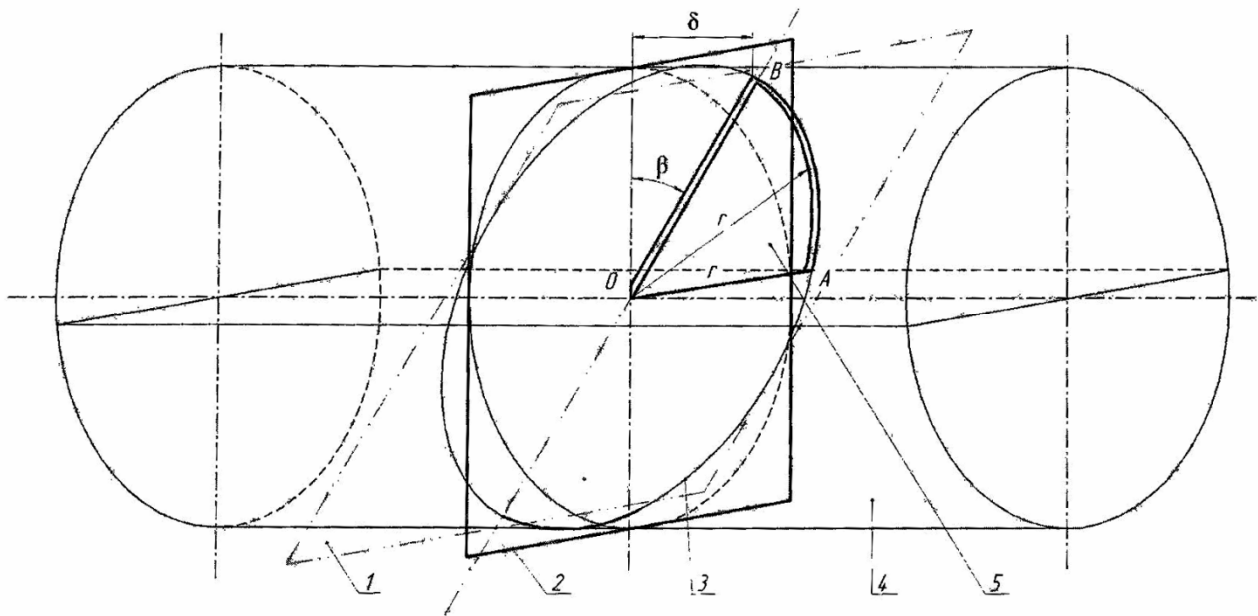
Рисунок 1 – Схема для определения геометрических параметров лопастей 1 – наклонная плоскость; 2 – плоскость вращения малой полуоси; 3 – эллипс; 4 – цилиндр; 5 – лопасть; \beta – начальный угол отклонения большой полуоси; \delta – ширина захвата Р.О.Д.; r – радиус основания цилиндра; OA = r = a – радиус основания цилиндра; OB = b – большая полуось эллипса.
