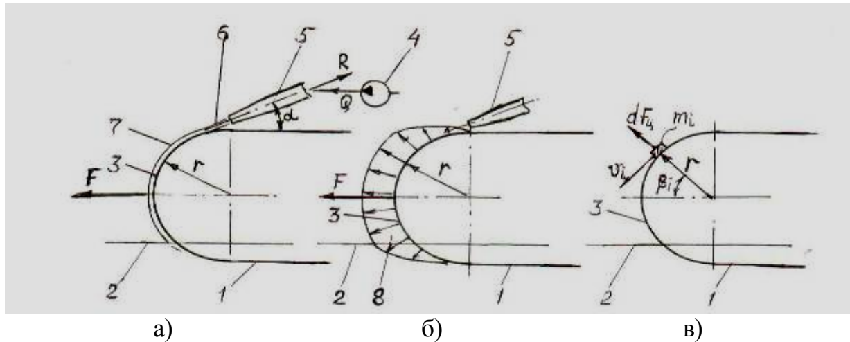
Рисунок 1 - Действие струи воды на сопло сверху-сзади на наружную цилиндрическую поверхность
