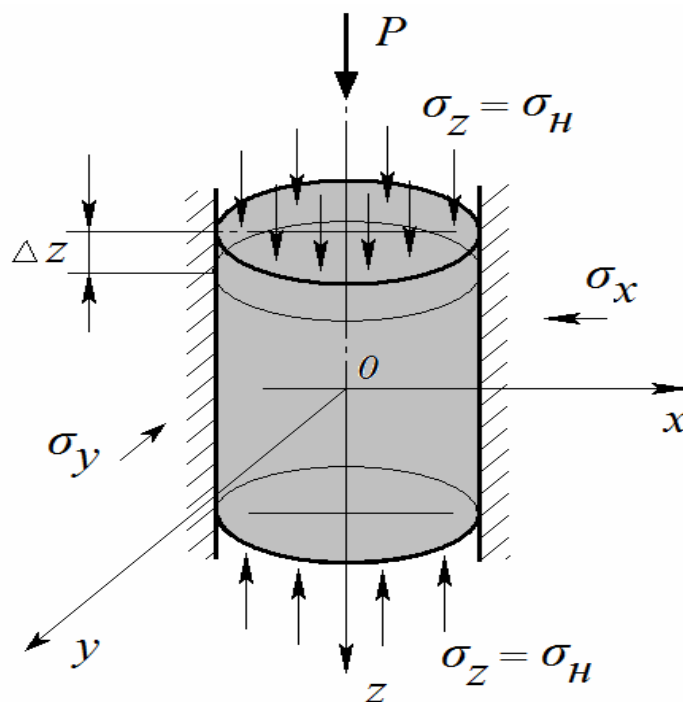
Рисунок 1 - Схема уплотнения лакированной смеси в замкнутом объеме
