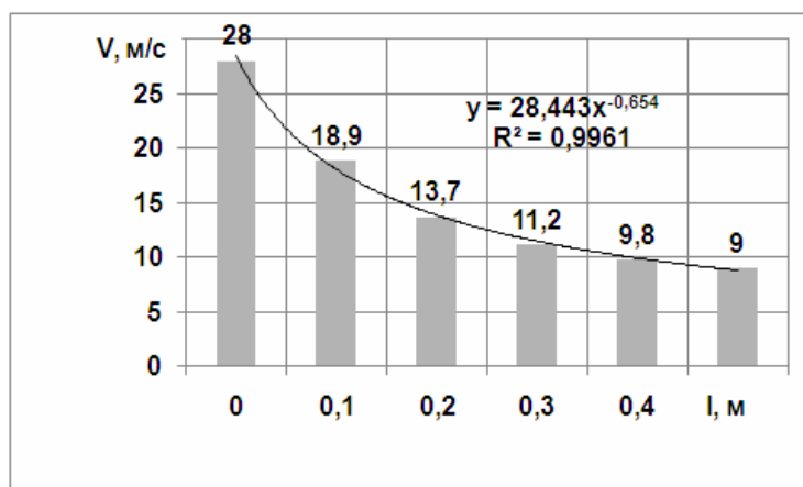
Рисунок 1 – Зависимость скорости V воздушного потока от расстояния l
