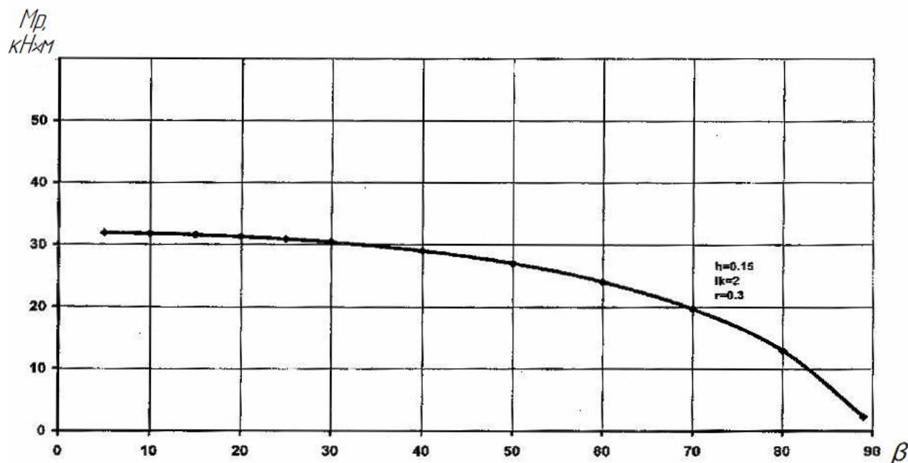
Рисунок 5 - Зависимость момента сопротивления резанию от угла отклонения большой полуоси эллипсовидной лопасти
