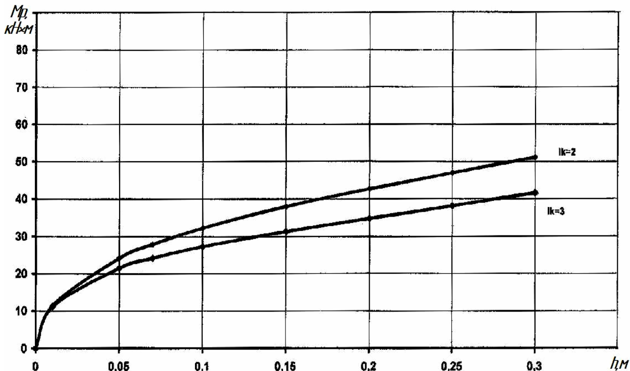
Рисунок 3 - Зависимость момента сопротивления резанию от глубины обработки почвы
