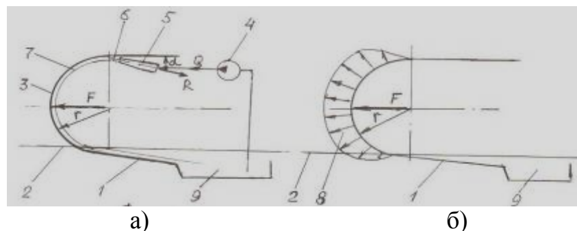
Рисунок 2 - Действие струи воды снизу-сзади на внутреннюю цилиндрическую поверхность
