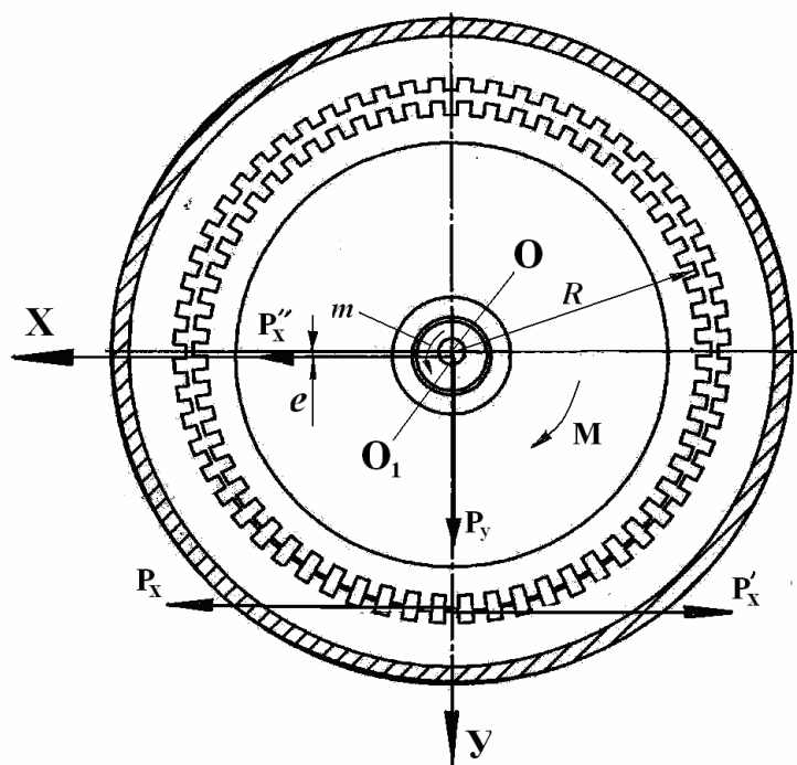
Рисунок 2. Силы, действующие между элементами механической передачи
