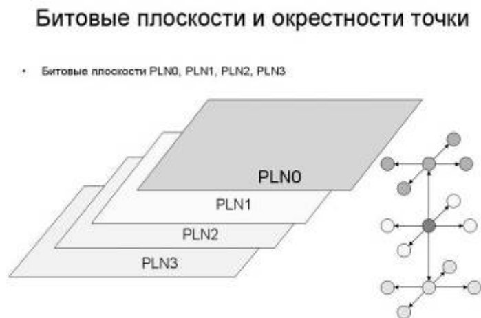
Рисунок 1 - Архитектура клеточного автомата
