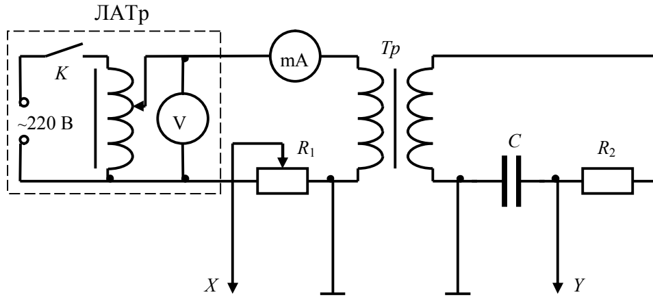
Рисунок - 2. Схема экспериментальной установ-
