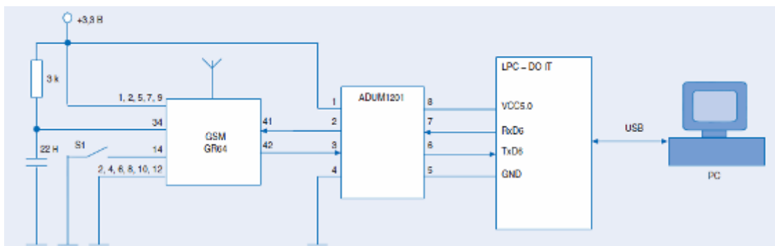
Рисунок 3 - Схема подключения GSM-модуля к оценочному комплекту.
