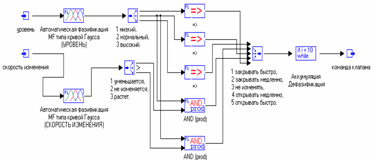
Рисунок 4 - Внутренняя структура блока управления
