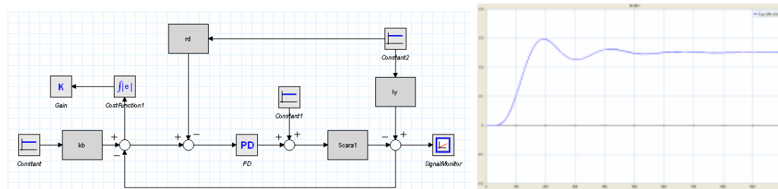
Рисунок 6 - Определение параметров PD-регулятора методом комбинированной коррекции
