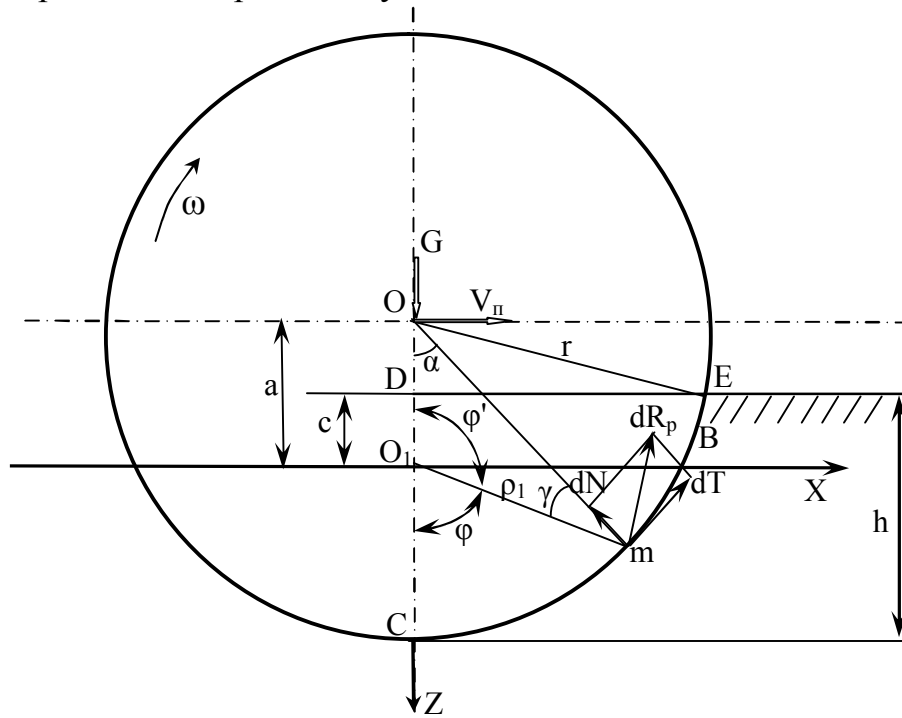
Рисунок 1 – Схема к определению элементарной реакции резания
