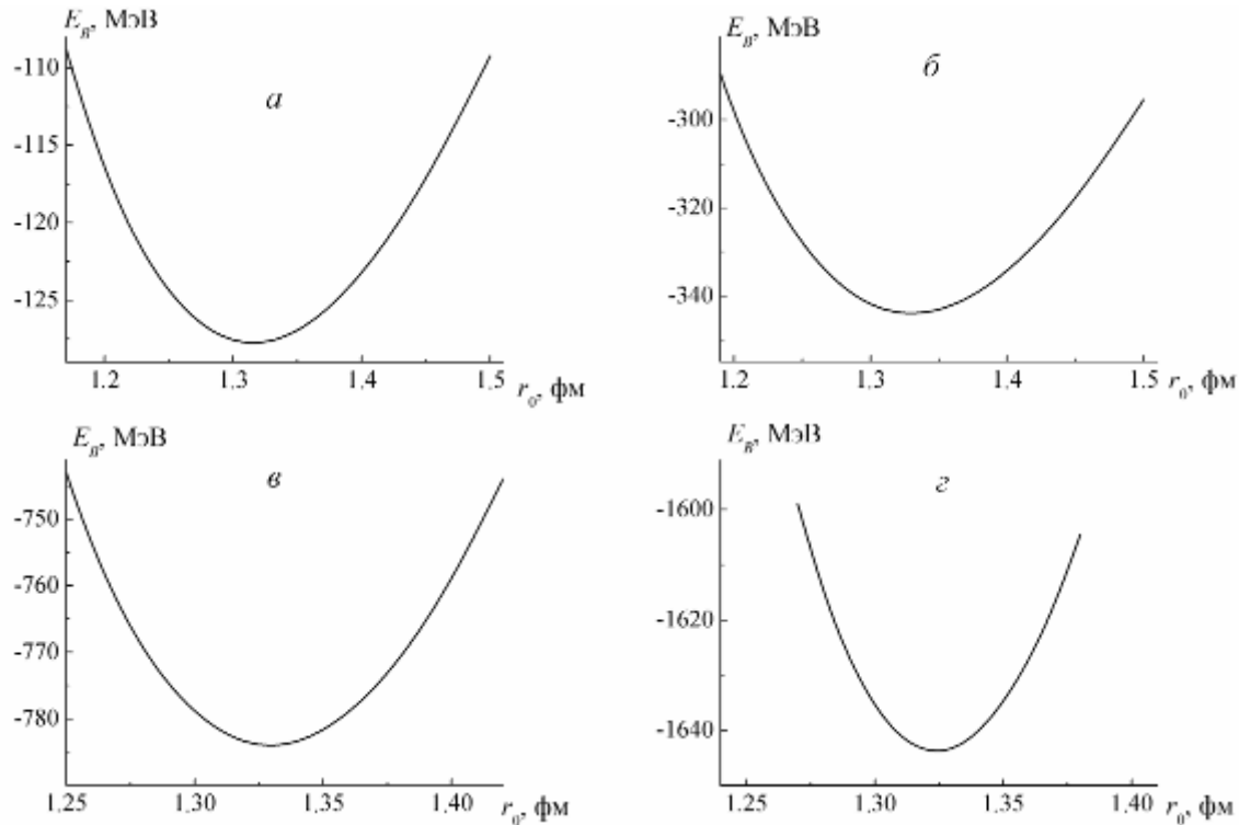
Рисунок 2 - Зависимости энергии основного состояния E_B(r_0) для ядер ^{16}\text{O} (а), ^{40}\text{Ca} (б), ^{90}\text{Zr} (в), ^{208}\text{Pb} (г)
