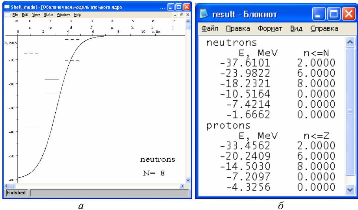
Рисунок 1 - Пример построения на экране монитора для ядра ^{16}\text{O} схемы расположения уровней с графиком потенциала (1) для нейтронов (а) и выходной файл с энергиями уровней E и числом нуклонов n на всех уровнях не выше данного (б). Заселенные нуклонами уровни показаны сплошными отрезками, незаполненные – штриховыми [4].
