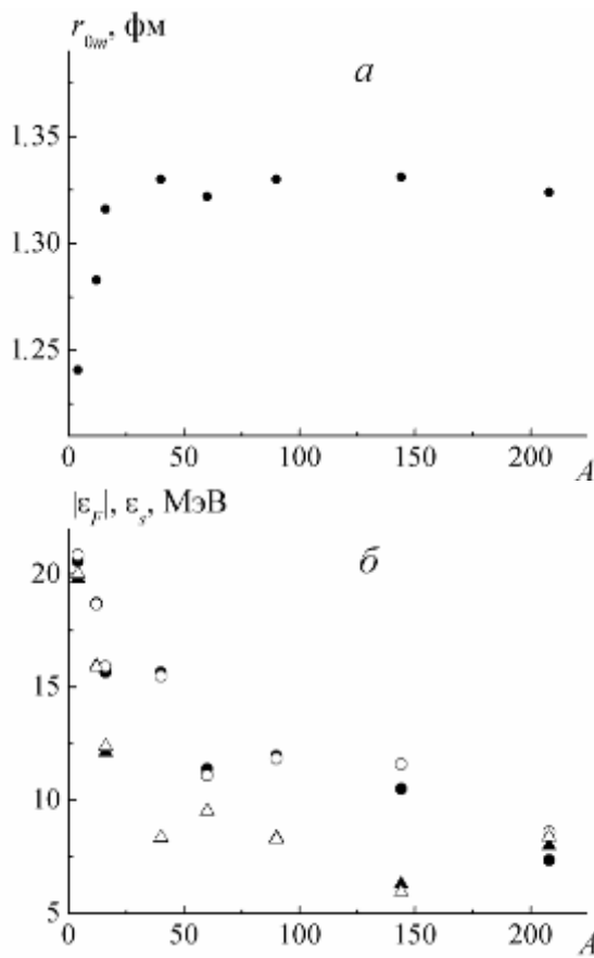
Рисунок 3 - Зависимости от массового числа A значений r_{0m} (a) и уровней Ферми – самых верхних заполненных нейтронных |\varepsilon_F^{(n)}| (○) и протонных уровней, |\varepsilon_F^{(p)}| (Δ) в сравнении с энергиями отделения от некоторых сферических четно-четных ядер нейтрона \varepsilon_s^{(n)} (●) и протона \varepsilon_s^{(p)} (▲) (б).
