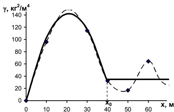
Рисунок 2 - Экспериментальная и теоретическая (по квадратичной с изломом модели) полувариограммы:
