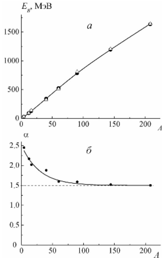
Рисунок 4 - a – Энергии связи E_B некоторых сферических четно-четных ядер: точки – экспериментальные данные, сплошная линия – сглаживающая кривая, треугольники – расчет с учетом (8); б – зависимость параметра \alpha от массового числа (точки) с графиком зависимости (8) (сплошная линия).
