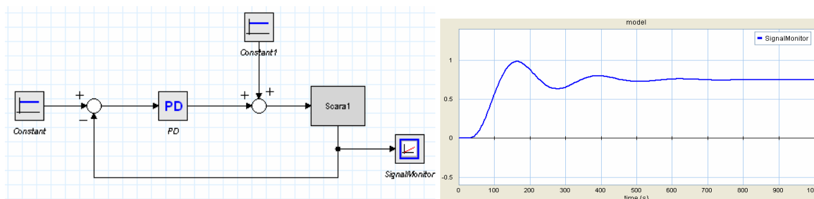
Рисунок 3 - Моделирование отдельного контура управления системы позиционирования
